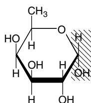
fucose
